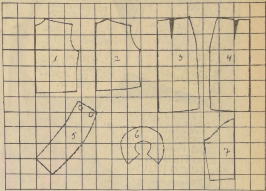
Molde del traje de dos piezas presentado en Ventana de la Moda, para talla 44 a escala de 10 cms. 1—Mitad delantero. 2—Mitad espalda. 3—Mitad delantero falda. 4—Mitad espalda falda. 5—Mitad pieza de cintura al sesgo. 6—Cuello. 7—Mitad de manga.
