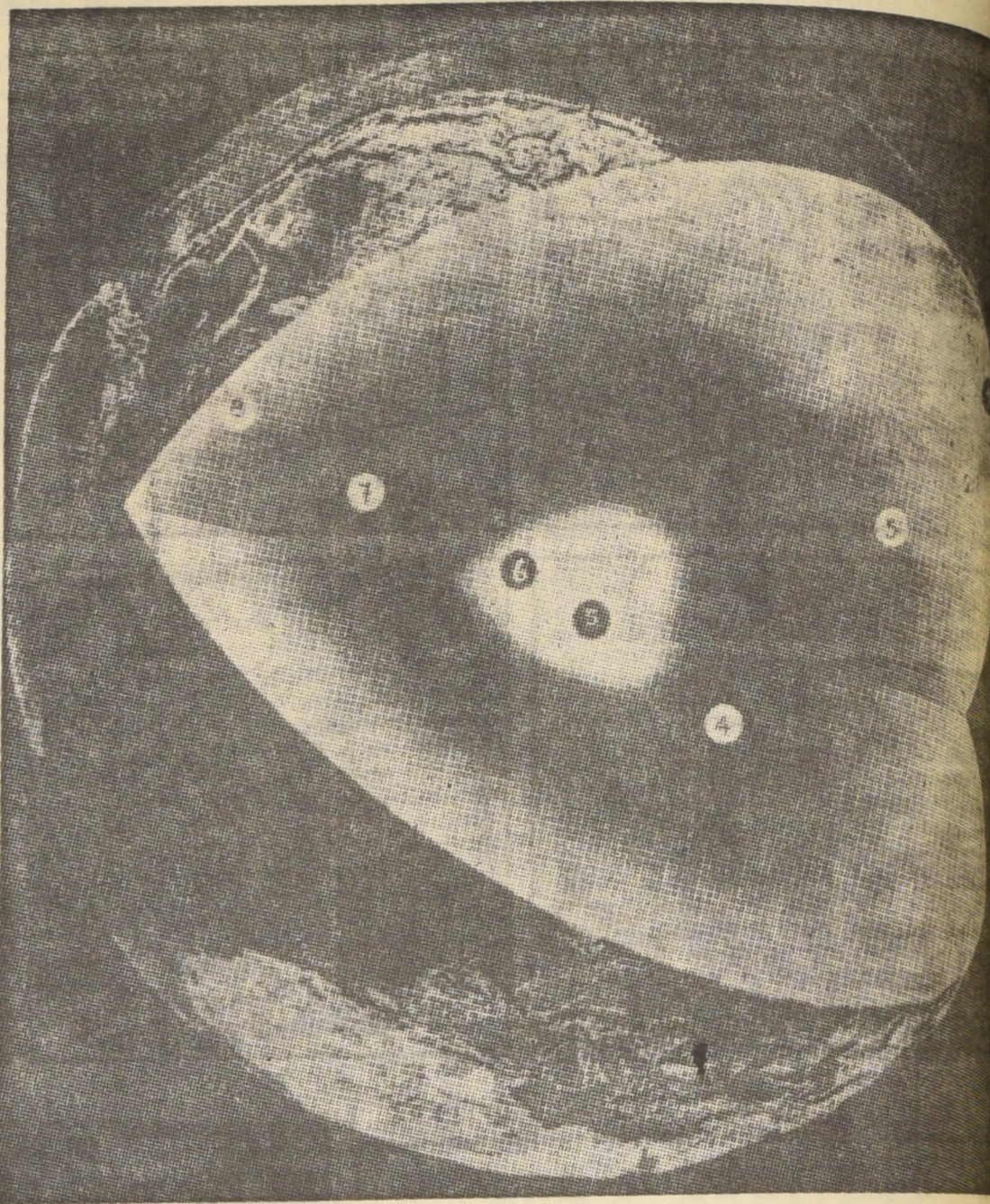
En esta disección de la Tierra, de acuerdo a un dibujo de "El Correo de la Unesco", aparecen descripciones siguientes: (1) CORTEZA. El espesor de la corteza de la tierra varía considerablemente; en el fondo del océano puede llegar con mucho a cinco kilómetros, y en los continentes oscila treinta y dos kilómetros. Actualmente se llevan a cabo planes de perforación de la corteza para llegar al manto.— (2) MOHO. La vertiente o "Discontinuidad de Mohorovicic" es el límite entre la corteza y el manto.— (3) MANTO. Se extiende desde la corteza terrestre hasta el núcleo. Se cree que es sólido y ligeramente plástico, que esté al rojo blanco, y que lo forman rocas diferentes de las de la corteza y más densas que éstas. La densidad del manto aumenta con la profundidad.— (4) NUCLEO EXTERNO. Se cree que sea una masa de hierro líquido al rojo blanco. La condición de líquido está dada por la conducta de las ondas sísmicas transver sales, que no pueden llegar a recorrerlo.— (5) NUCLEO INTERNO. Se ha señalado la posibilidad de que dentro del núcleo externo, que es líquido, exista otro interno en el centro, y que éste sea sólido.— (6) El Núcleo Interno podría tener una extensión de 1.270 kilómetros.— (7) El núcleo externo podría extenderse hasta 2.200 kilómetros.— (8) El manto podría tener una extensión de 2.900 kilómetros.
