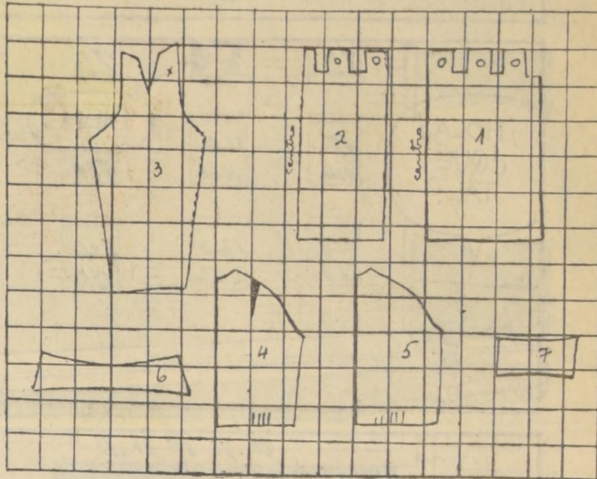
Molde del abrigo de niña, presentado en Ventana de la Moda. El molde va a escala de 10 cm., para 10 años.
