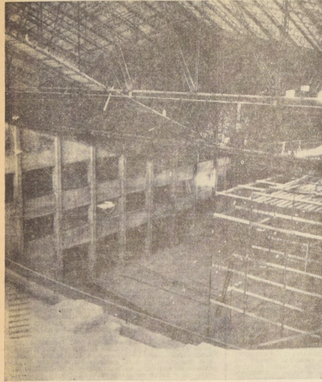
EL ARMAZON INTERIOR de la techumbre, en la parte superior, luciendo su impresionante estructura de fierro, y abajo el ring-side o cancha para basquetbol, tenis, pimpon, voleibol, equitación, etc. Al fondo, parte de la platea baja. La capacidad total del estadio será de 10 mil personas, cómodamente sentadas.
