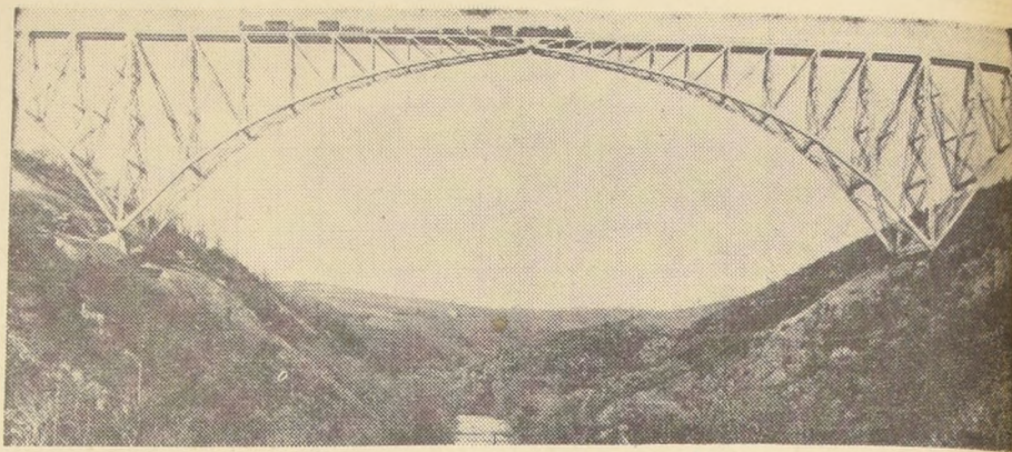
Viaducto de Garabit, construido por Eiffel.
