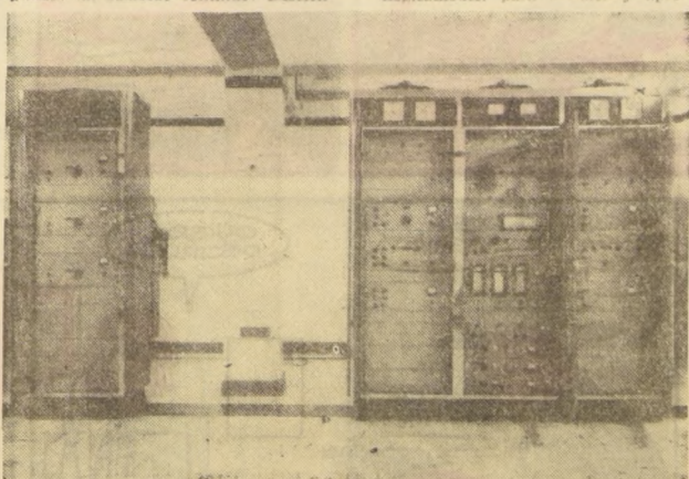
Aspecto del triple reloj electrónico de cuarzo. Llegó a Chile en 1964. A la izquierda aparece el "corazón" del instrumento, donde tres láminas de cuarzo, al vacío y 46° de temperatura, vibran un millón de veces por segundo. Precisión horaria: cienmilésimo de segundo.
