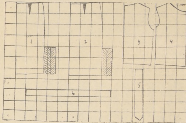
Molde a escala de 10 cms. para talla 44 del conjunto presentado en Ventana de la Moda: 1.—Mitad espalda falda. 2.—Mitad falda delantera. 3.—Mitad jumper espalda. 4.—Mitad jumper delantero. 5.—Patita colocada desde el hombro hasta más abajo de la cintura, para pasar el cinturón. 6.—Cinturón.
