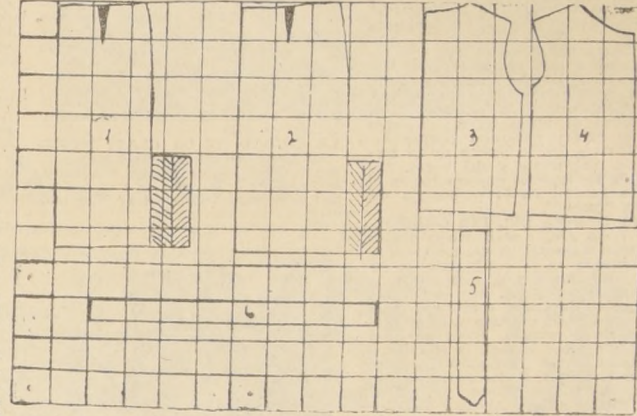
Molde a escala de 10 cms. para talla 44, del conjunto presentado en Ventana de la Moda: 1.—Mitad espalda falda. 2.—Mitad falda delantera. 3.—Mitad jumper espalda. 4.—Mitad jumper delantero. 5.—Patita colocada desde el hombro hasta más abajo de la cintura, para pasar el cinturón. 6.—Cinturón.
