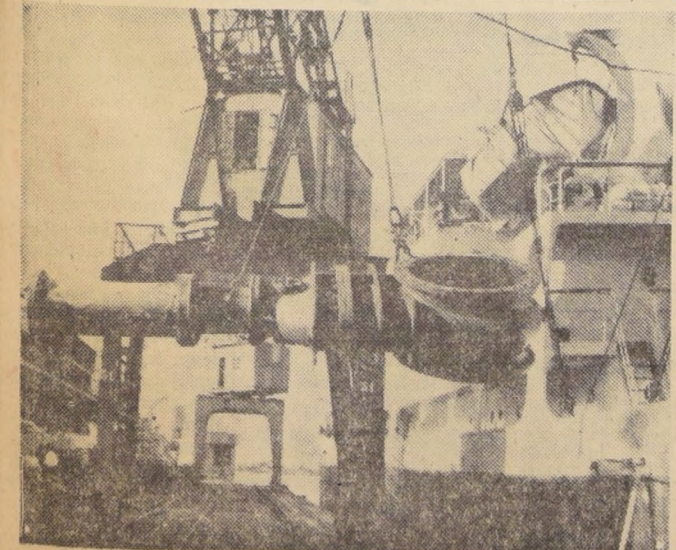
Centro toneladas pesa una de las válvulas gigantes que ayer fue desembarcada del vapor "Cienfuegos" y que será instalada en la nueva Planta de Filtros "Las Vizcachitas", que construye la Empresa de Agua Potable de Santiago, en el camino a El Volcán, a 25 kilómetros del centro de la capital. Estos elementos son los primeros que llegan al país procedentes de Inglaterra, con cargo al préstamo que por 5 millones 125 mil dólares concedió el Banco Interamericano de Desarrollo al servicio de utilidad pública mencionado.
