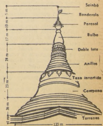
Estructura de la pagoda
