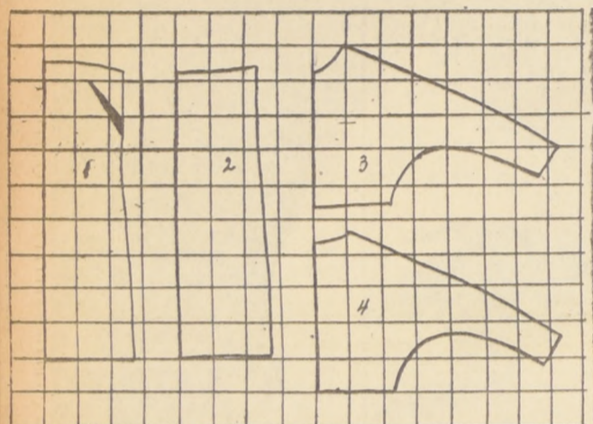
Molde a escala de 10 cm., para talla 44, del vestido presentado en Ventana de la Moda. 1.—Mitad delantero parte interior. 2.—Mitad espalda parte interior. 3.—Mitad delantero blusa tul. 4.—Mitad espalda blusa.
