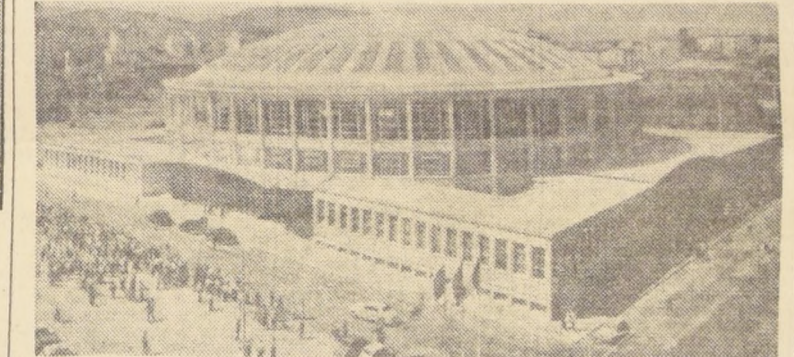
EL PALACIO DE LOS DEPORTES DE BOLONIA, una de las obras de mayor interés arquitectónico en su especie, construido en el año 1956. Arquitecto Rocatelli y Valle, Ingeniero Francisco Allegra.
