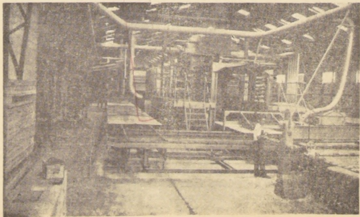
He aquí, en primer plano, la Canteandora y, al fondo, la prensa, de la Fábrica de MASISA, en Valdivia.
