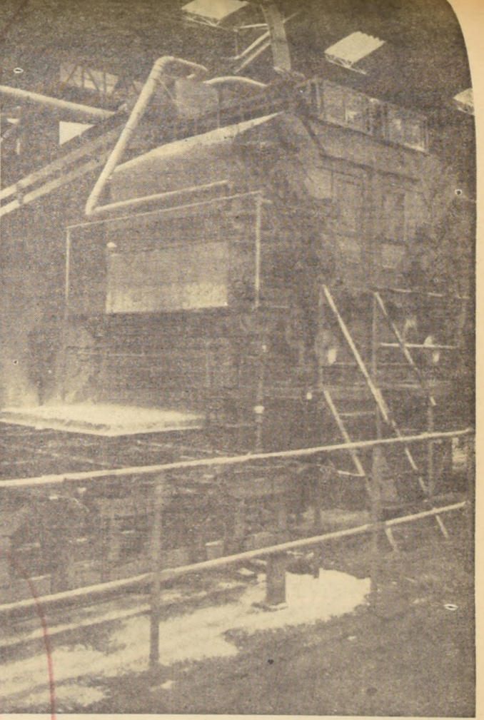
MAQUINA conformadora de la placa o esparcidora de las astillas. Es un moderno equipo, que fuera montado por técnicos alemanes.
