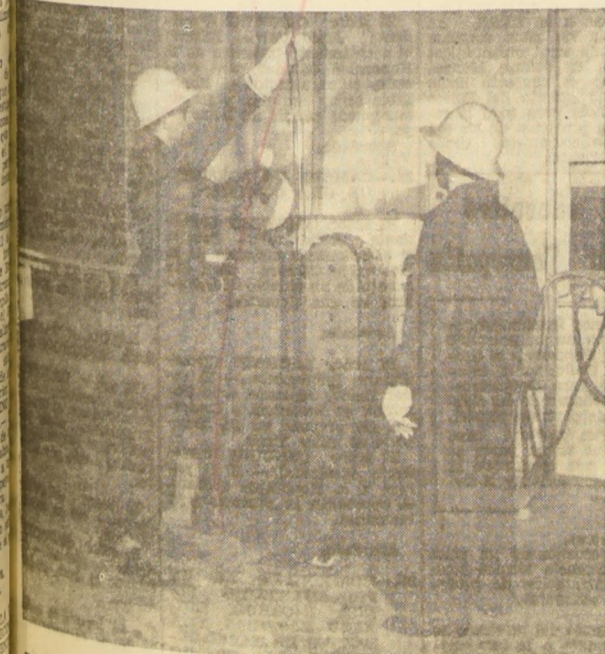
Esta unidad eleva el tubo continuo que entrega el equipo de extrusión y alimenta una máquina cortadora a mecheros, que da la dimensión exacta a los tubos.
