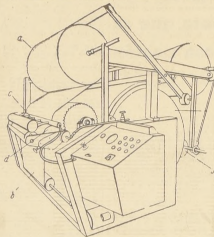
MAQUINA DE FORRADO, con llama abierta, para láminas de poliuretano esponjado. a) Banda de material esponjado; b) Banda textil; c) Mecheros desplazables; d) Cilindros de forrado; e) Tambor de secado; f) Producto acabado.
