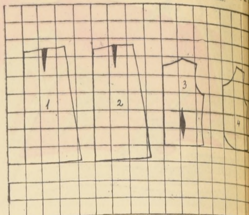
Molde a escala de 10 cm. para talla 44 del traje presentado en Ventana de la Moda. 1.— Mitad delantera falda. 2.— Mitad espalda falda. 3.— Mitad espalda chaqueta. 4.— Mitad delantera chaqueta.
