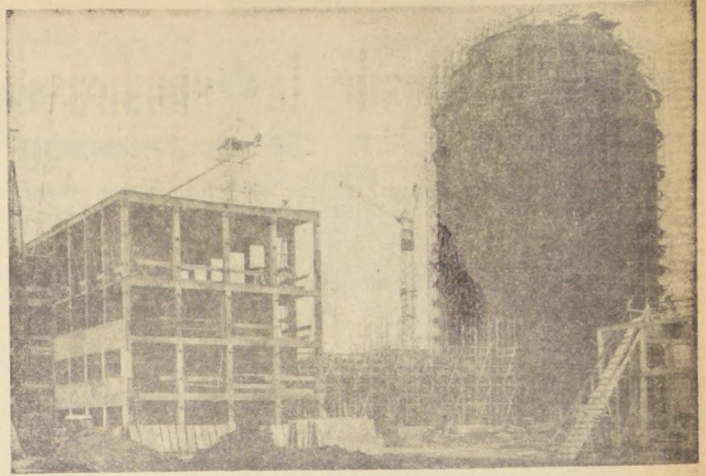
LA CENTRAL DE ENERGIA ATOMICA de Gundremmingen, en el Valle del Danubio, en el sur de Alemania, ya merece algunos superlativos. Cuando esté terminada en 1966, será la mayor planta de reacción del continente europeo. Se habrán invertido, hasta entonces, 350 millones de marcos. Producirá 260 megavatios de energía, lo que corresponde a 340.000 caballos vapor. En sólo seis meses se construyó el casco de presión del reactor. Parece una columna gigantesca, de 50 m. de altura, un símbolo moderno en un paisaje idílico donde hasta ahora casi no hay empresas industriales.
