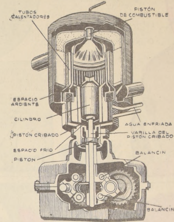
LA EXTRASA geometría del motor Stirling, a propulsión romboidal, y con dos pulsos de energía en cada revolución.
