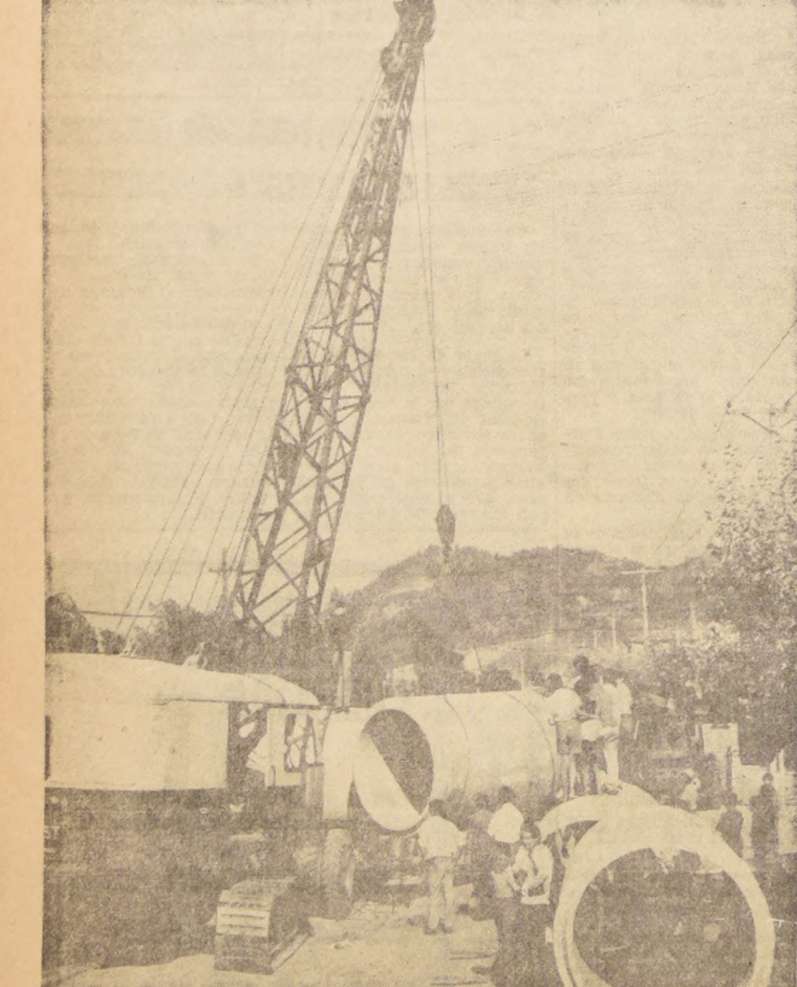
CIGANTESCOS TUPOS de cemento armado, de 1,80 metro de diámetro, canalizarán las aguas del canal La Punta, de las comunas de Renca y Conchalí. Los trabajos de desvío y entubamiento de las aguas demorarán dos meses, y en esta labor trabajarán unos 40 obreros. El costo total de las obras ha sido calculado en $ 140.000, incluyendo la colocación de cercos de seguridad en los puntos más peligrosos. El canal La Punta se ha hecho tristemente célebre debido a la sucesiva muerte de niños en sus turbulenta aguas, motivo que impulsó a las autoridades de Gobierno a buscar una rápida solución a este grave problema.— EN EL CRABADO, los inmensos tubos que aprisionarán las aguas del canal La Punta.
