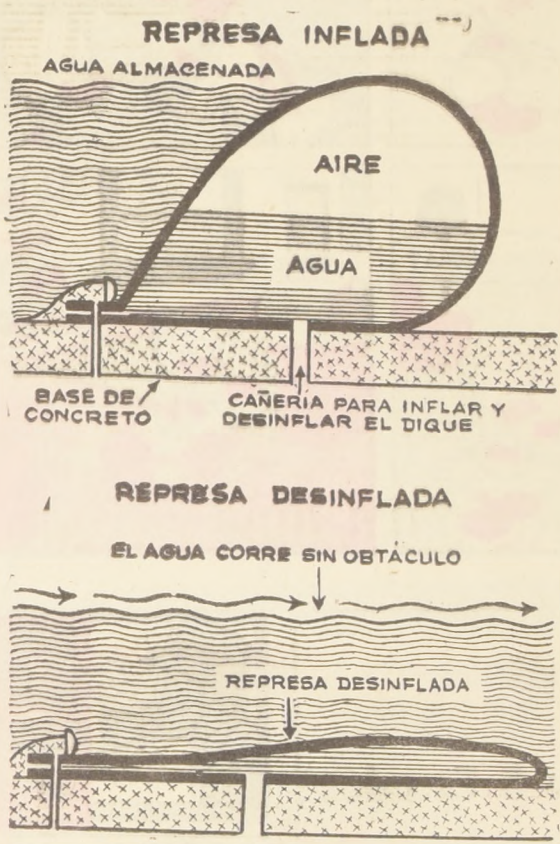
La represa FABRIDAM, en Sunbury, se infla para contener las aguas del rio Susquehanna. Pero es desinflada en la época de las inundaciones primaverales, para no debilitar la resistencia de los muros.
