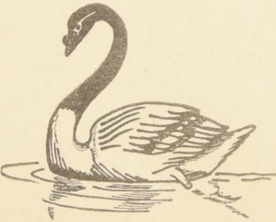
El Cisne de Cuello Negro (Cygnus Melancoryphus, Molina.).
