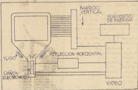
En la nueva televisión en colores, con tubo plano, los circuitos del barrido de imágenes son diferentes, como se observa en el esquema adjunto.
