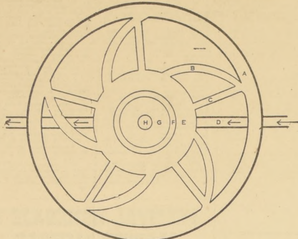
A.— Pista principal. B.— Cambio de dirección de alta velocidad. C.— Carretero para la salida. D.— Acceso de automóviles (subterráneo, bajo las pistas y rampas. E.— Estacionamiento de aviones. F.— Edificio del terminal del aeropuerto. G.— Estacionamiento de autos y jardines. H.— Torre de control y radio-faro.
