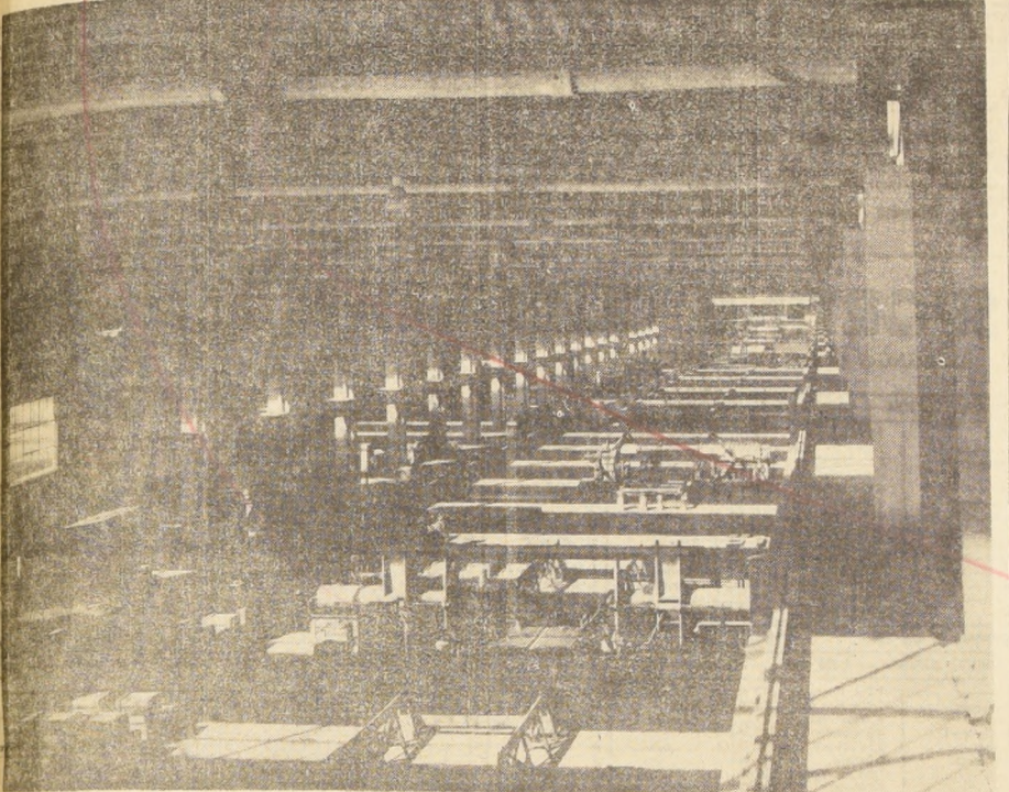
Pruebas de presión. Los tubos de asbesto-cemento prueban soportando a grandes presiones de agua, bajo el control de inspectores del Instituto de Ensayos de Materiales de la Universidad de Chile. En el grabado, los tubos llegan, uno a uno, a la máquina de presión.
