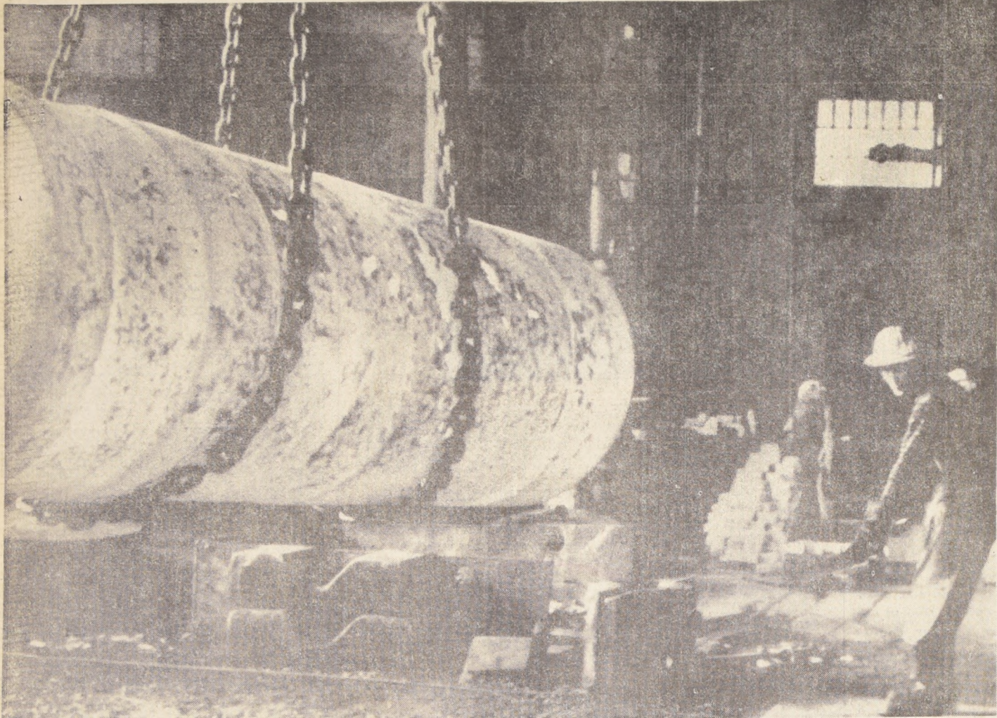
Acaba de ser fundido en el mayor lingote de titanio del mundo. Con sus diez toneladas de peso, su longitud de tres metros y el diámetro de un metro, alcanza el acualidad de la capacidad técnica de un moderno horno de fundición. Titanio, un elemento blanco argentino, existe en la naturaleza exclusivamente en combinación con oxígeno y hierro. Después de un complicado proceso de fundición, que en un lingote de diez toneladas dura dos días, desde la primera fundición hasta el enfriamiento, se obtiene el material bruto granuloso, la llamada esponja titánica. Este metal maravilloso, sumamente resistente e incorrosible, va conquistando cada vez más campos de aplicación. Su poco peso específico —tiene solamente la mitad del peso del acero— y su elevada gama de cargas, lo hacen atractivo particularmente para la industria de aviación y de astronáutica. El empleo de remaches de titanio en lugar de los corrientes remaches de aluminio permitieron reducir el peso sin carga de un avión de transporte en 3,5 toneladas. Desempeña un papel importante el titanio, asimismo, para la industria automovilística, por ejemplo, para bielas y otras piezas del motor. Así se consiguió aumentar la potencia de un coche de deporte de 210 a 270 km/h. El proceso de fundición ahora logrado constituye el resultado de una técnica de elaboración para titanio seguida desde hace 15 años.
