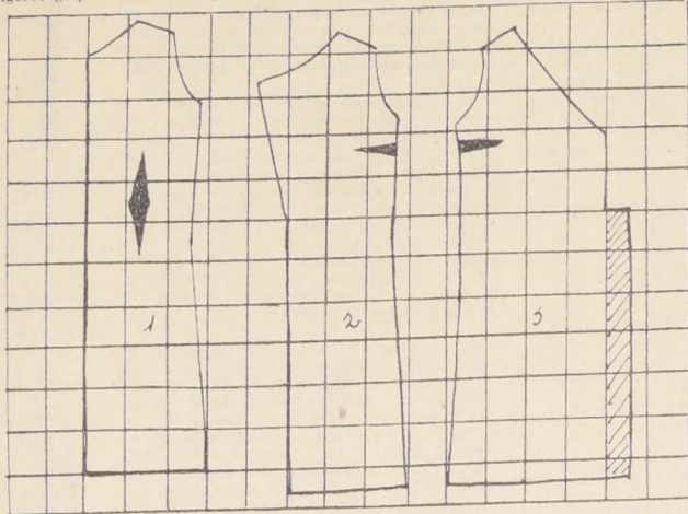
Molde a escala de 10 cms., para talla 46, del vestido presentado en Ventana de la Moda: 1.- Mitad espalda; 2.- Delantero izquierdo; 3.- Delantero derecho.
