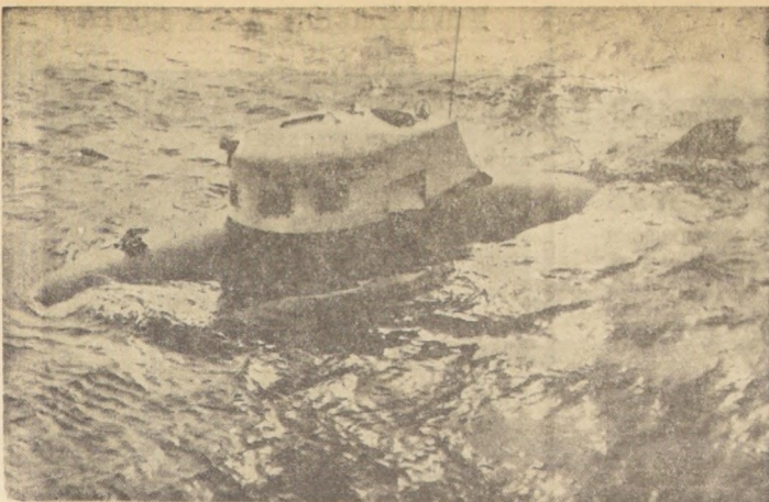
Submarino de bolsillo quieren comprar los rusos. El "Star III" es un pequeño submarino para dos tripulantes. Tiene ocho metros de eslora, pesa diez toneladas, lo mueve un motor eléctrico de 7 1/2 caballos y vale US$ 900.000. Ha sido diseñado principalmente para fines de exploración científica, y posee tres "brazos" que pueden levantar cualquier cosa, desde un lápiz hasta algo que pese 200 libras. Los rusos están muy interesados en comprar uno a la General Dynamics que lo construye, pero parece que no autorizará el negocio el Gobierno norteamericano.
