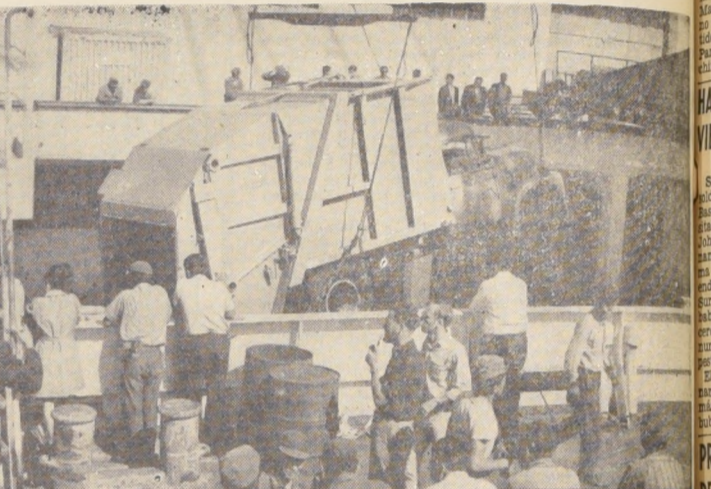
VALPARAISO.— El barco danés "Nordholm" arribó desde Nueva Orleans con 23 camiones de aseo para Santiago, marca Pak Mor, de fabricación norteamericana, los que forman parte de un total de 100 encargados por el Municipio de la capital. En el grabado aparece un aspecto del desembarco en el espigón de atraque de estos grandes camiones.
