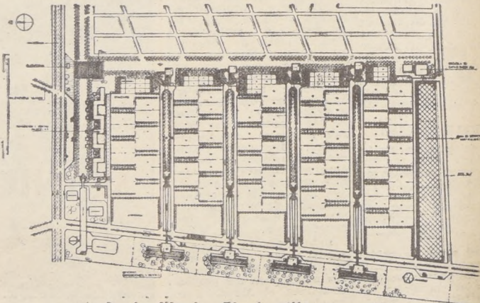
PARQUE INDUSTRIAL EN LA REINA. PLANTA GENERAL. ESCALA 1:500. UNIVERSIDAD CATOLICA DE CHILE. CIUDAD PROYECTISTA. ARQUITECTO: ENRIQUE BROWNE C.
