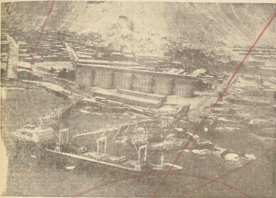
Sistema mecanizado de embarque de salitre a granel en el puerto de Tocopilla; consta de seis silos de almacenamiento, correa transportadora y brazo mecánico de carguío.
