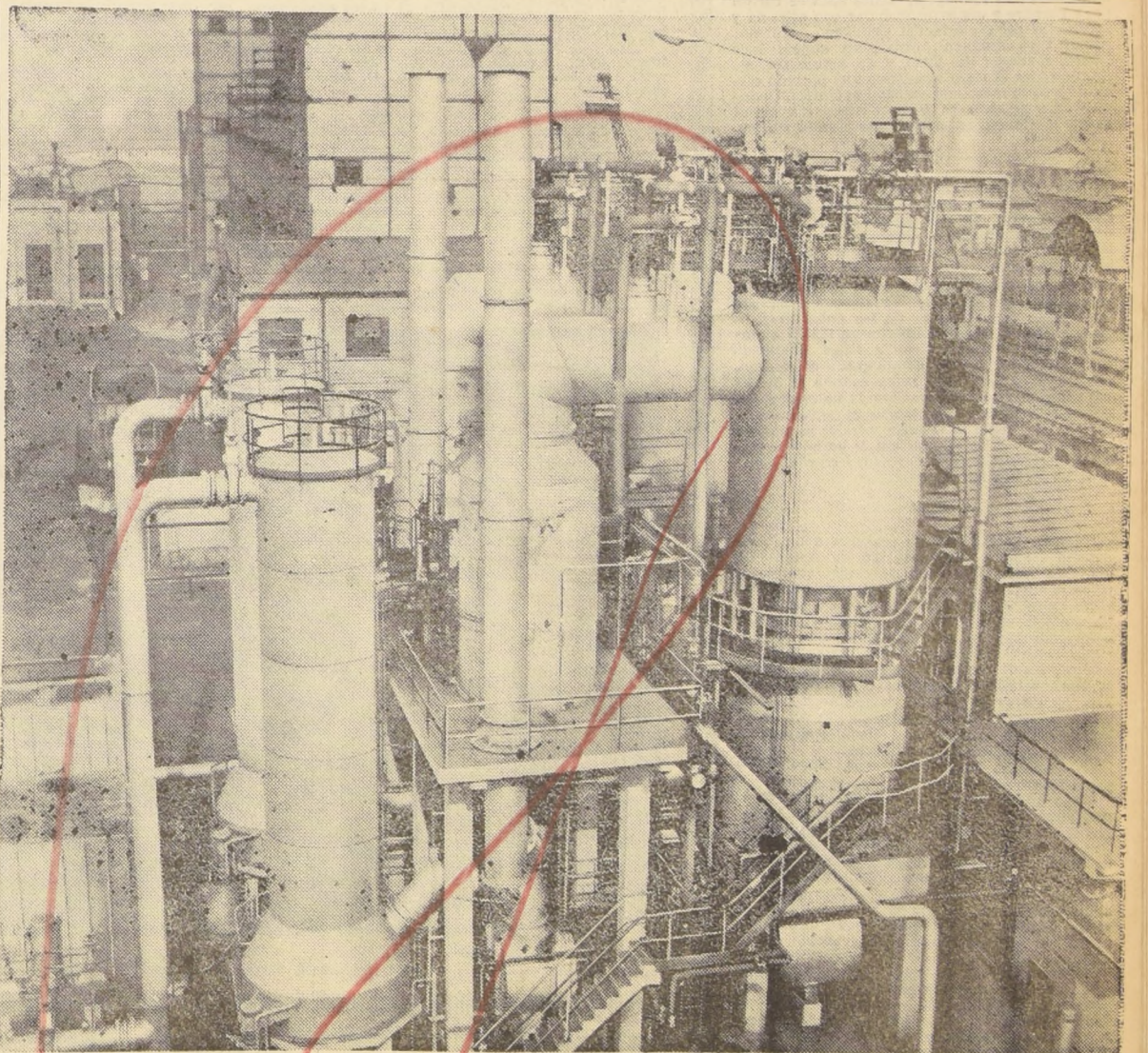
(Vista parcial de la planta de Cracking Catalítico instalada en la Fábrica San Jorge).
