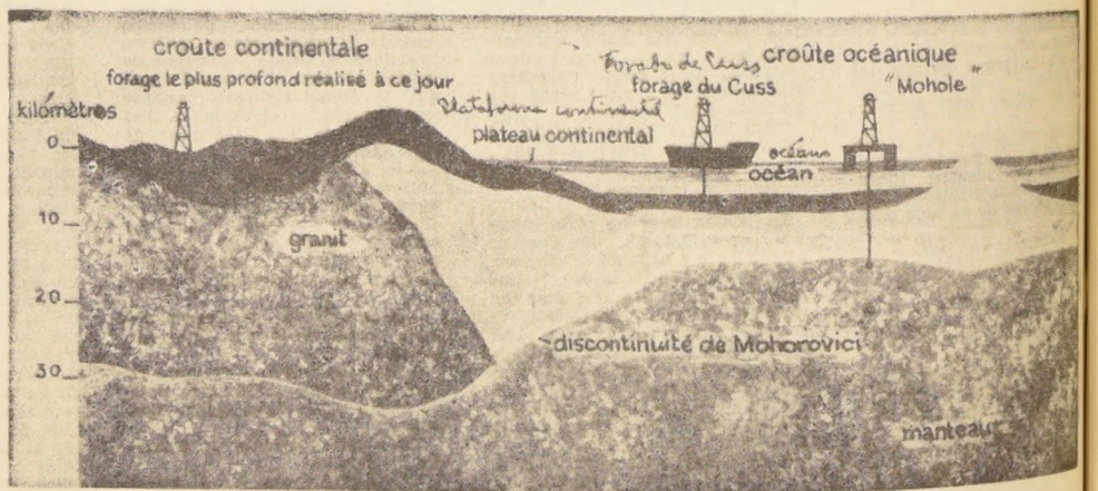
Corte esquemática de la corteza, del "Moho" y del Manto terrestre con alusión a las perforaciones en el océano y en tierra firme.
