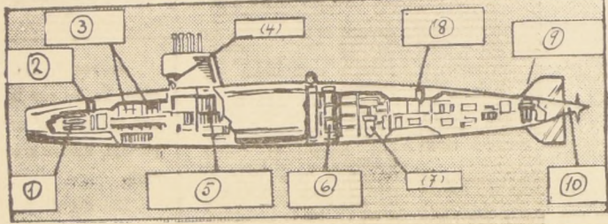
DISPOSITIVO INTERIOR DEL "REDOUTABLE"— (1) Cámara de torpedos— (2) Escotilla de salvamento— (3) Alojamiento y comedor de la tripulación— (4) Escotilla de acceso— (5) Puesto central de navegación y operaciones— (6) Tubo lanza-cohetes— (7) Reactor— (8) Escotilla de salvamento de la popa— (9) Motor eléctrico auxiliar— (10) Timón de profundidad.
