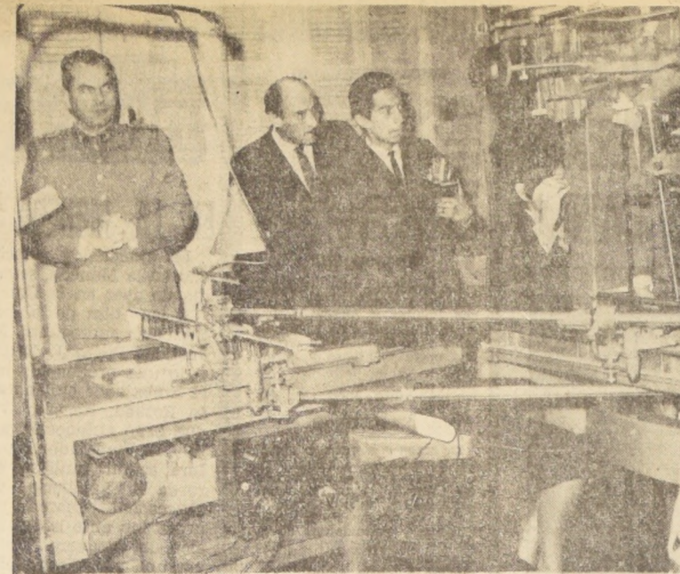
El operador por medio de la visión estereoscópica obtiene nitidamente la real y exacta forma del terreno y puede trazar en el papel de dibujo la planimetría completa, encuadrada en los valores en ella estampados y la altimetría por medio de controles mecánicos de manera de lograr la mayor precisión en el trazado de las curvas de nivel. Todo lo que observa el operador de restitución lo va dibujando en la hoja que ya mantiene preparada sobre el tablero metálico a su espalda.
