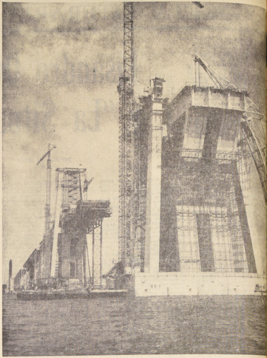
Estructuras metálicas sobre el lago Maracaibo.
