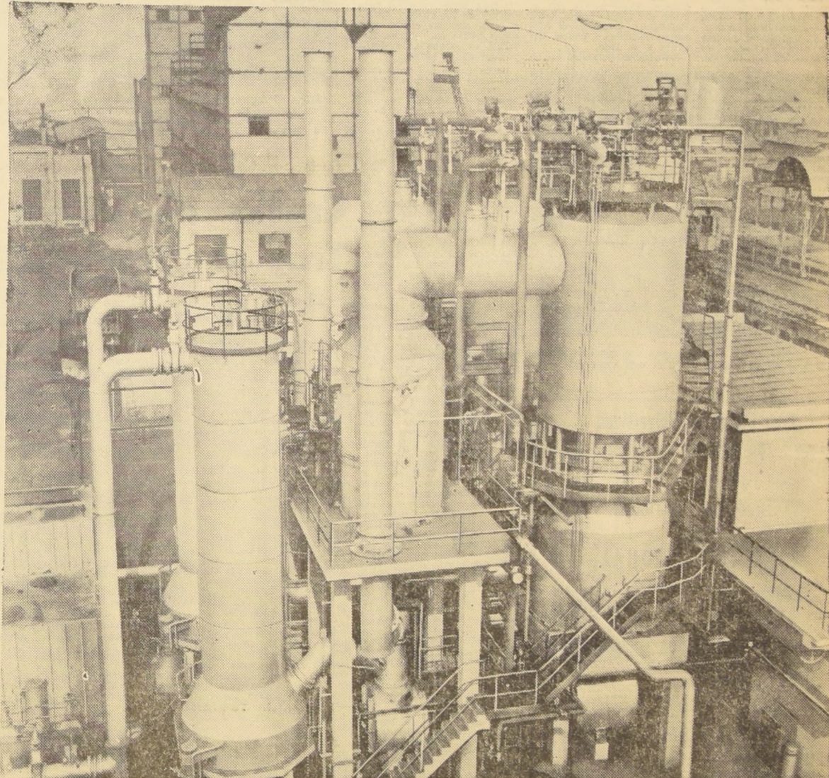
(Vista parcial de la planta de Cracking Catalítico instalada en la Fábrica San Borja).
