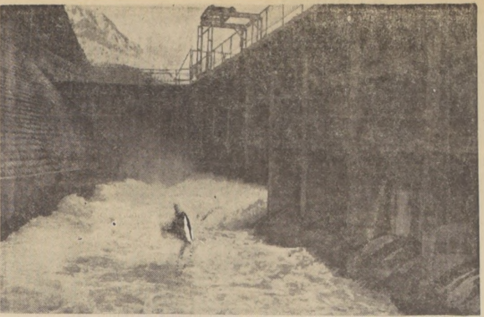
TALCA. BOCATOMA ARMERILLO DEL SISTEMA MAULE NORTE. — 250 kilómetros en canales comprende el Sistema de Riego Maule Norte, de los cuales están terminados ya cerca del 45%, y que con el Embalse Digua permitirán el riego total de las provincias de Linares y Talca. Ambas obras las realiza el Ministerio de Obras Públicas, dentro de la Alianza para el Progreso. En el grabado, una vista de la bocatoma Armerillo del Sistema Maule Norte.
