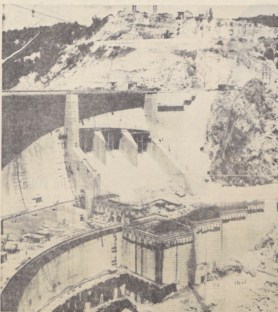
El Ministro de Minería, Alejandro Hales, visitó ayer la construcción de la Planta Hidroeléctrica de Rapel, que está en sus fases finales de instalación y empezará a entregar energía al país en los próximos seis meses. Acompañaron en esta visita al Ministro, el vicepresidente de la CORFO, Raúl Sáez; el Gerente General de la ENDESA, Renato Salazar, y otras altas personalidades. Las explicaciones fueron dadas en el terreno mismo, por el ingeniero jefe, a cargo de estas obras, Santiago Bonhomme. En el grabado, una parte del gigantesco muro de contención, de forma circular que tiene 111 metros de alto, y que es una de las obras más importantes realizadas en toda la historia de la Ingeniería civil del país.
