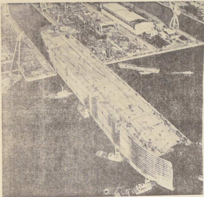
Esta curiosa vista aérea muestra el proceso de construcción del mayor buque actualmente existente en el mundo, un petrolero de 300.000 toneladas, la cual se está realizando en un astillero japonés en Yokohama. La proa, montada en sección aparte, será unida al resto de la estructura posteriormente. (Foto UPI)
