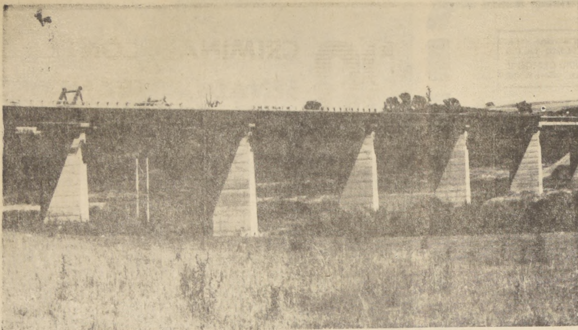
En su visita a la provincia de Valdivia, el Ministro de Obras Públicas y Transportes, Sergio Ossa Pretot, inaugura hoy el puente Río Bueno, construido en el programa de la Alianza para el Progreso. Esta moderna obra de ingeniería tiene una estructura de concreto armado con vigas de hormigón. Su largo es de 325 metros, y su ancho de ocho, a Osorno y Valdivia
