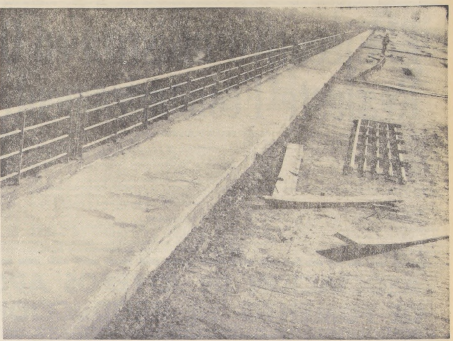
El puente Mapocho, situado en la localidad de El Paico, cuyos trabajos de construcción se encuentran en sus fases finales, significa un gran avance en el complejo caminero de doble vía que unirá a Santiago y Melipilla. Esta obra de ingeniería tiene una estructura de hormigón de 462 metros de largo por 20 de ancho. Posee dos pistas de 8 metros cada una y calzadas laterales para peatones de dos metros de ancho. Representa una inversión de 5 millones de escudos.
