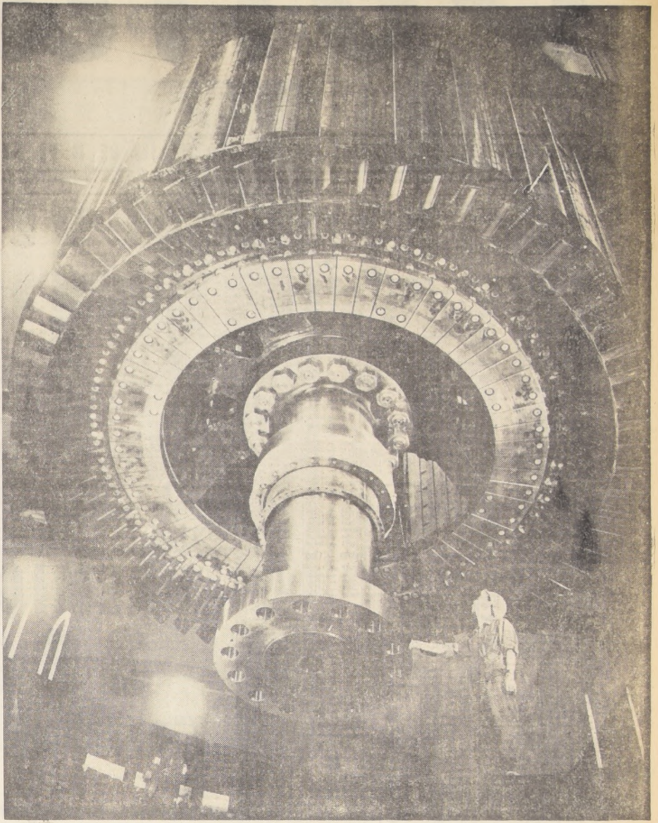
La estatura de un hombre normal, da la idea de las dimensiones de este rotor para turbina, construido por la industria eléctrica pesada.
