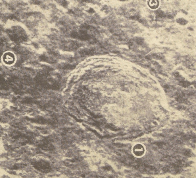
MOSCU.— Fotografía de la superficie lunar captada por el navio lunar soviético "Zond-6", y dada a la publicidad por científicos espaciales. Los cráteres visibles y numerados son: 1, Hermanos Vavilov; 2, Lowell; 3, Eves; 4, Van Goo. (Radiofoto UPI.)
