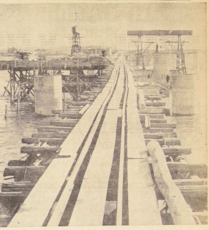
En Concepción se construye aceleradamente el nuevo puente sobre el Bio-Bio. Tendrá una longitud de 1.400 metros que lo convertirá en el más largo de Chile y uno de los más largos de América Latina, cuando quede terminado en febrero de 1970. Este nuevo puente, que se construye dentro de la Alianza para el Progreso, tendrá un costo total de unos 15 millones de dólares y en su financiamiento se emplea un crédito del Banco Interamericano de Desarrollo. Sus dos pistas de circulación, de ocho metros de ancho cada una, tendrán capacidad para un tráfico de 48 mil vehículos diarios. El puente visto actualmente en uso no soporta el paso de camiones o buses con un peso superior a las 12 toneladas y resulta estrecho para el intenso movimiento de vehículos.
