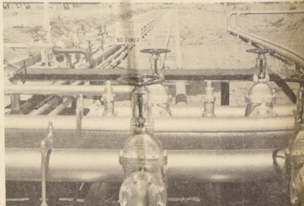
En los principales centros urbanos la ENAP está construyendo depósitos de almacenamiento de combustible, que permiten bajar los costos de transporte y ofrecer un mejor abastecimiento. En el grabado, tuberías de un depósito que lleva el combustible a los estancos.
