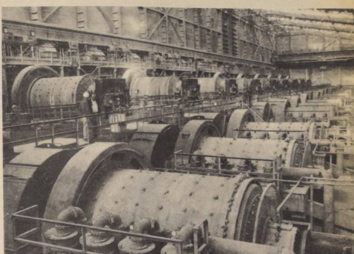
CHILE es el segundo productor de cobre del mundo. Sus reservas incalculables lo ubican en condiciones altamente ventajosas frente a cualquier país competidor. En la foto: interior de la planta concentradora de Chuquibambilla.
