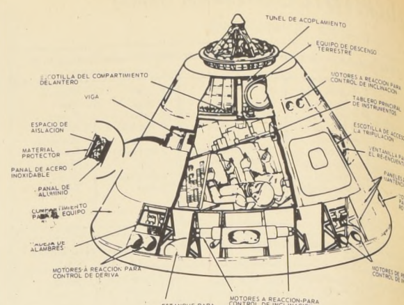
Este dibujo en corte muestra el interior del módulo de comando de la Apolo-11 en el que los tres astronautas regresarán hoy a la Tierra una vez cumplida su misión lunar.
