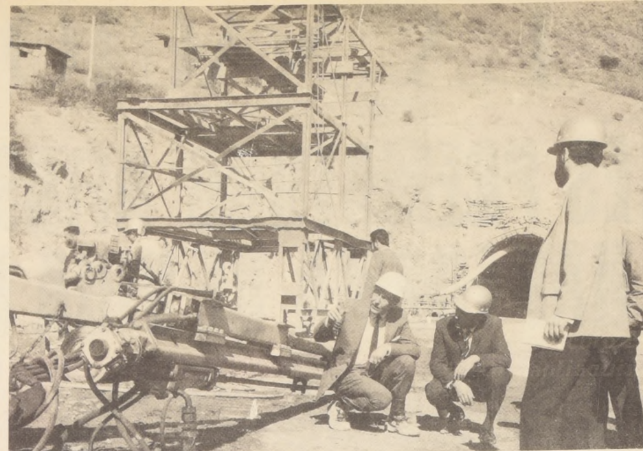
ESTA A PUNTO de alcanzarse el 50% de la perforación del túnel Lo Prado. Observan el trabajo el Ministro Ossa Pretet y el Intendente Jorge Kindermann.
