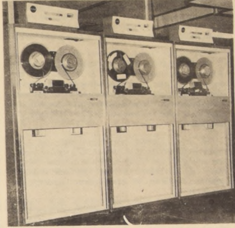
Vista de algunas de las unidades de cinta magnética, que forman parte del sistema de computación electrónica recién inaugurado.
