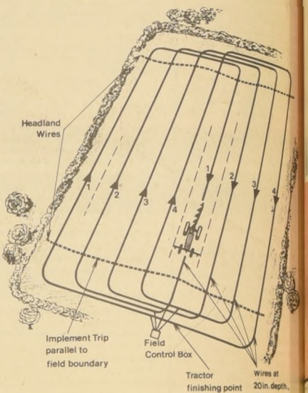
Colocación idónea de los alambres de dirección, que se entierran bajo el terreno para conducir al "Autotrak".
