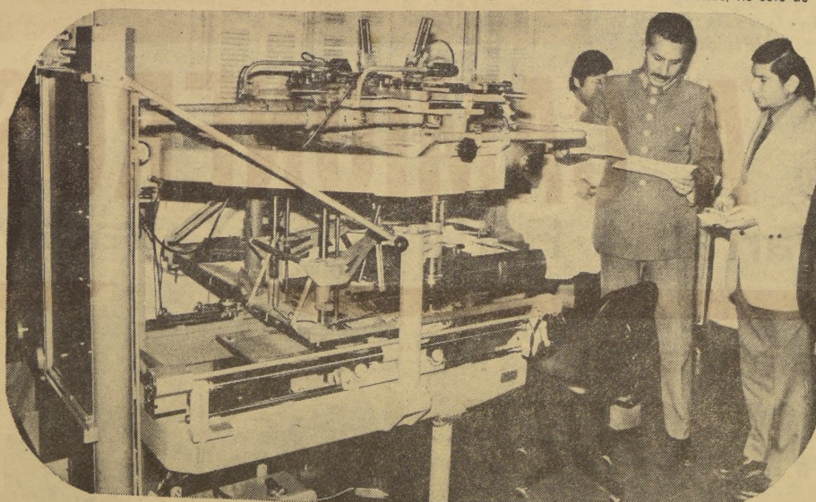
Una complicada máquina para Restitución de fotografías aéreas. El mayor Marcos García muestra los trabajos que están en ensayos.
