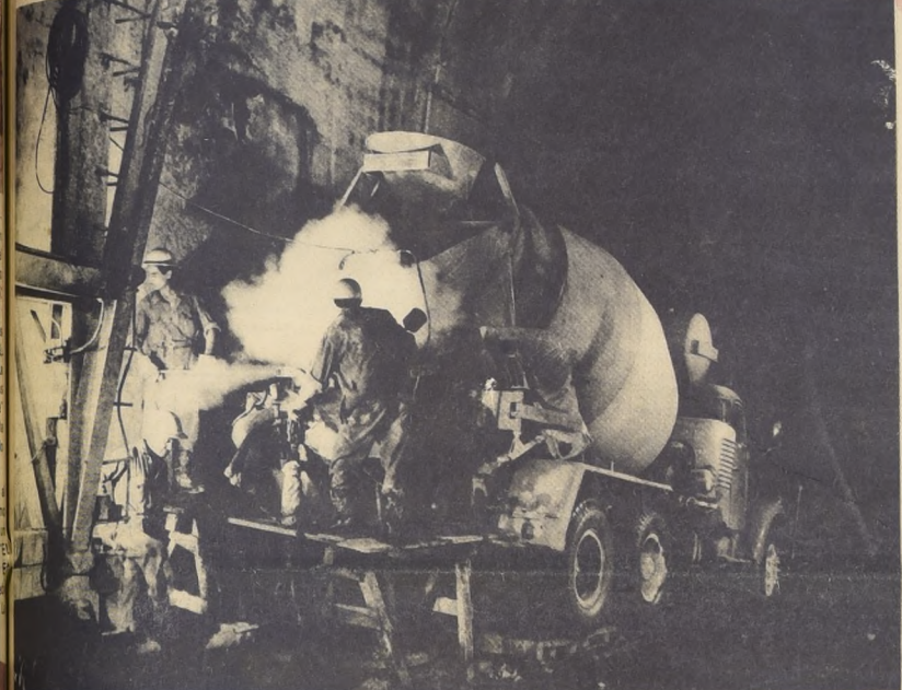
UNA "CONCRETERA" en plena labor durante las faenas de revestimiento del túnel "Lo Prado". Las medidas de seguridad y la proverbial laboriosidad del obrero chileno.
