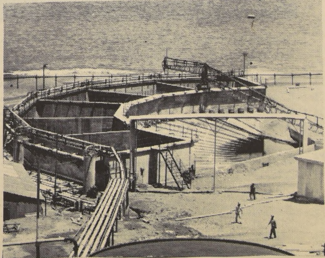
Estanques de lixiviación por percolación de la Planta "José Antonio Moreno" de ENAMI en Talca. Este plantel, construido y puesto en marcha por el actual gobierno, fue recientemente ampliado de 3.900 toneladas mensuales de minerales a 18.000 toneladas mensuales.
