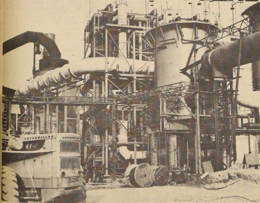
PLANTA ACIDO SULFURICO
