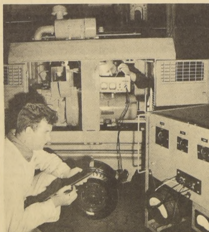
EQUIPOS MOVILES DE RADIO BRITANICOS. Destinados a la Dirección General de Investigaciones, una fábrica electrónica de Cinderford, Inglaterra, prepara 60 equipos generadores móviles para alimentar transmisores de radio. De ellos, 57 serán equipados con patines para su rápida instalación en cualquier lugar. Cada equipo está dotado de un motor Diesel Lister SR-1, que desarrolla 5 caballos de fuerza y va directamente conectado a un generador de 3 kilowatts. La maquinaria es cubierta totalmente de acero a prueba de situaciones climáticas. En el grabado, técnicos de la Compañía Hawker Siddeley someten a prueba de circuito uno de los equipos.
